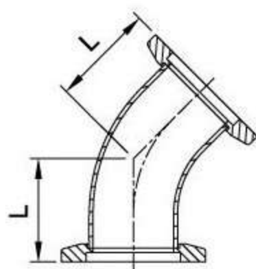
45° Elbow Flange
