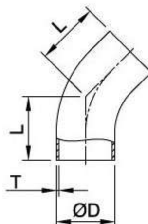
45° Long Elbow
