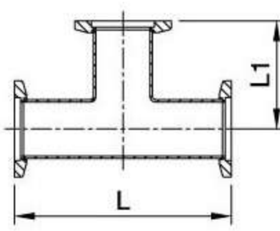
Tee Flange
