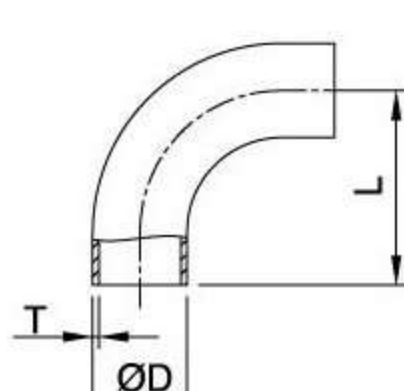
90° Long Elbow
