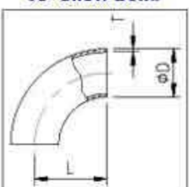
C.2WCL-90° Bend
