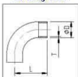
C.L2S-90° Bend
