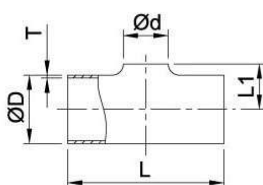
BS ETL Long Tee
